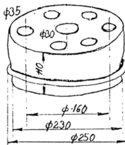
Ryc. 13. Drewniany tłok zaworowy (II 8)
