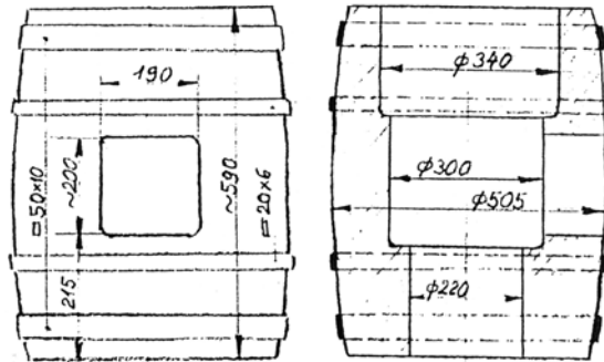
Ryc. 11. Korpus zaworu ssącego (II 3)
