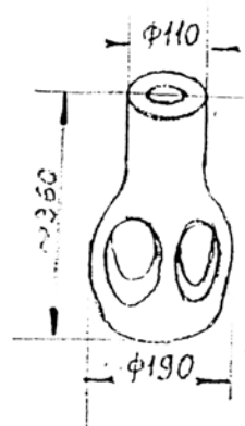
Ryc. 20. Drewniany kosz ssący (IV 7)
