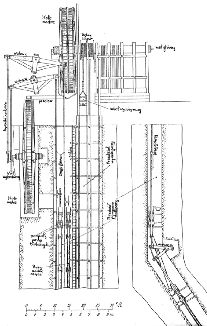
Ryc. 3. Projekt z 1783 r. instalacji napędowej do wydobywania wrobku rudnego i pomp wodnych dołowych zasilanej wodą powierzchniową dla kopalni rud cynowych Hundsrücken w Gierczynie.
