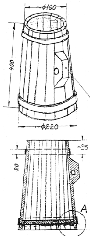
Ryc. 4. Drewniana konew czerpalna (I 2)
