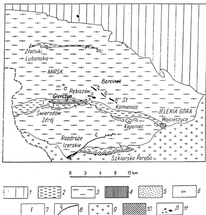
Ryc. 1. Występowanie surowców skalnych w okolicach Gierczyna: 1 – seria metamorficzna, 2 – łupki łyszczykowe, 3 – gnejsy, 4 – granaaty, 5 – leukogranity, 6 – grejzeny i utwory skałizowane, 7 – kwarcyty fluorytowe, 8 – żyły kwarcowe, 9 – granity, 10 – łupki kordierytowo-andaluzytowe, 11 – bazalty
