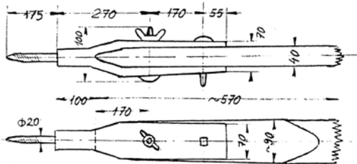
Ryc. 18. Złącze dwudzielne drąga głównego (III 2)
