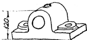
Ryc. 7. Łożysko oczkowe odlewane (I 6)
