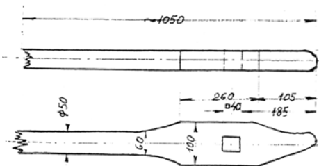
Ryc. 15. Fragment tłoczyska (II 12)
