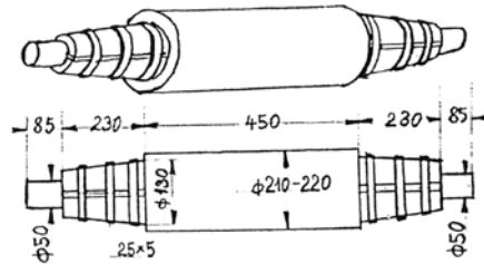
Ryc. 9. Wał – bęben (I 9)
