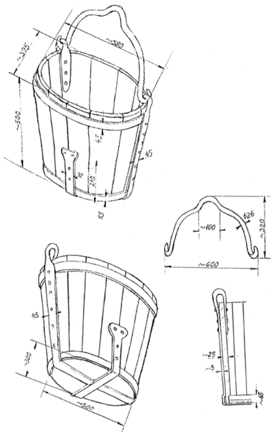
Ryc. 21. Kubeł drewniany (V 1)
