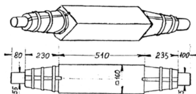
Ryc. 5. Wał drewniany (I 4)
