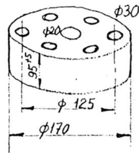
Ryc. 14. Drewniany tłok zaworowy (II 9)
