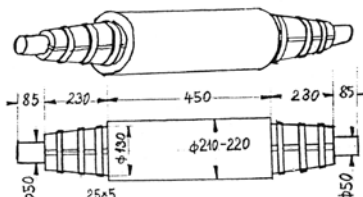
Ryc. 8. Wał – bęben (I 8)
