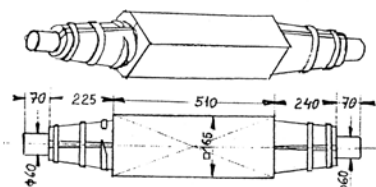
Ryc. 6. Wał drewniany (I 5)
