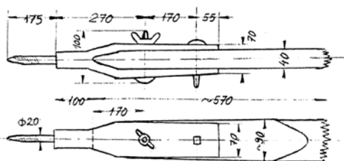
Ryc. 17. Trzpień kwadratowy z końcówką nagwintowaną (II 18)
