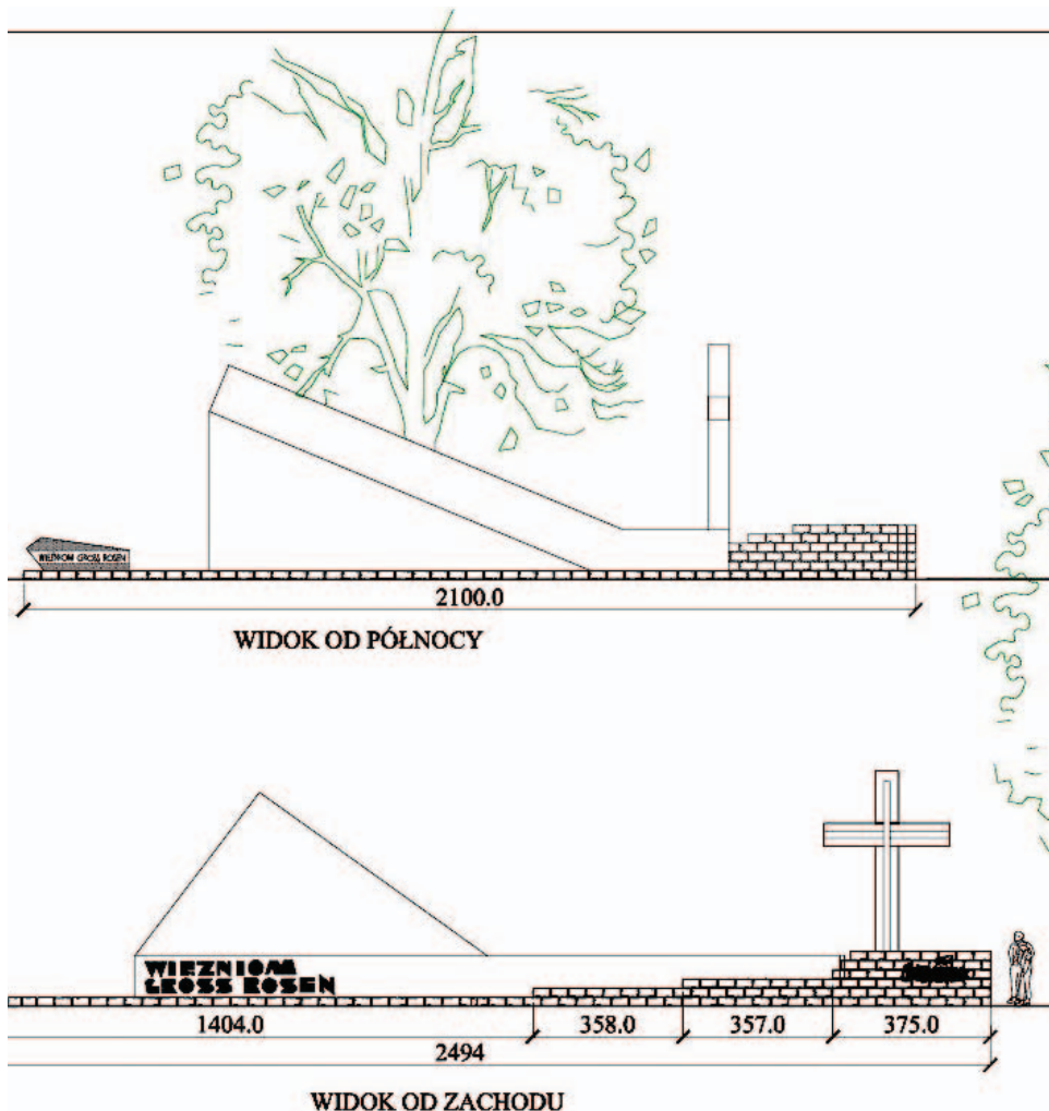
Projekt pomnika - widok od strony północnej i zachodniej
