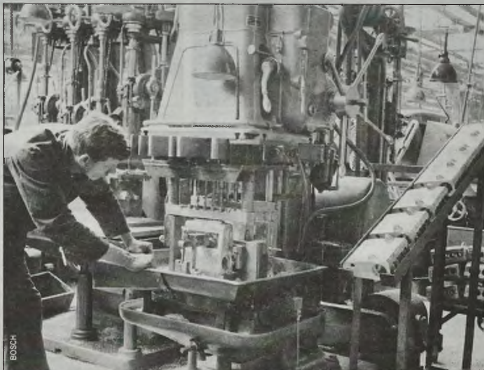
Produkcja pomp wtryskowych do silników wysokoprężnych - obróbka obudów w fabryce w Feuerbach w Niemczech, rok 1935
