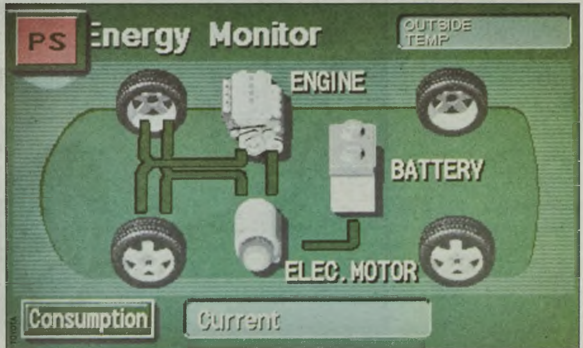
Wyświetlacz pokazuje rozkład siły przenoszonej przez silniki spalinowy i elektryczny na poszczególne osie
