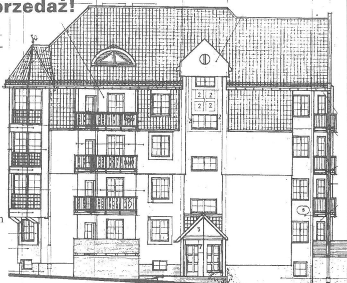
Luban, ul. Kopernika 7. Projekt elewacji bocznej
