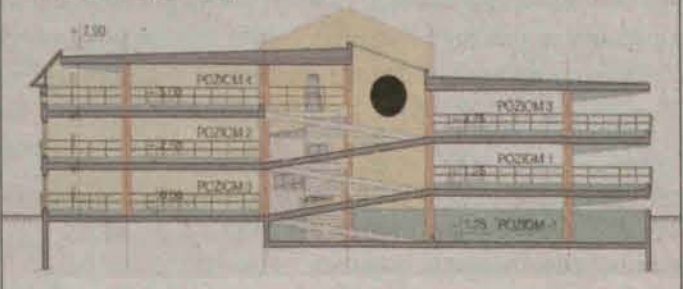
PRZEKRÓJ A - SKALA 1 : 100
