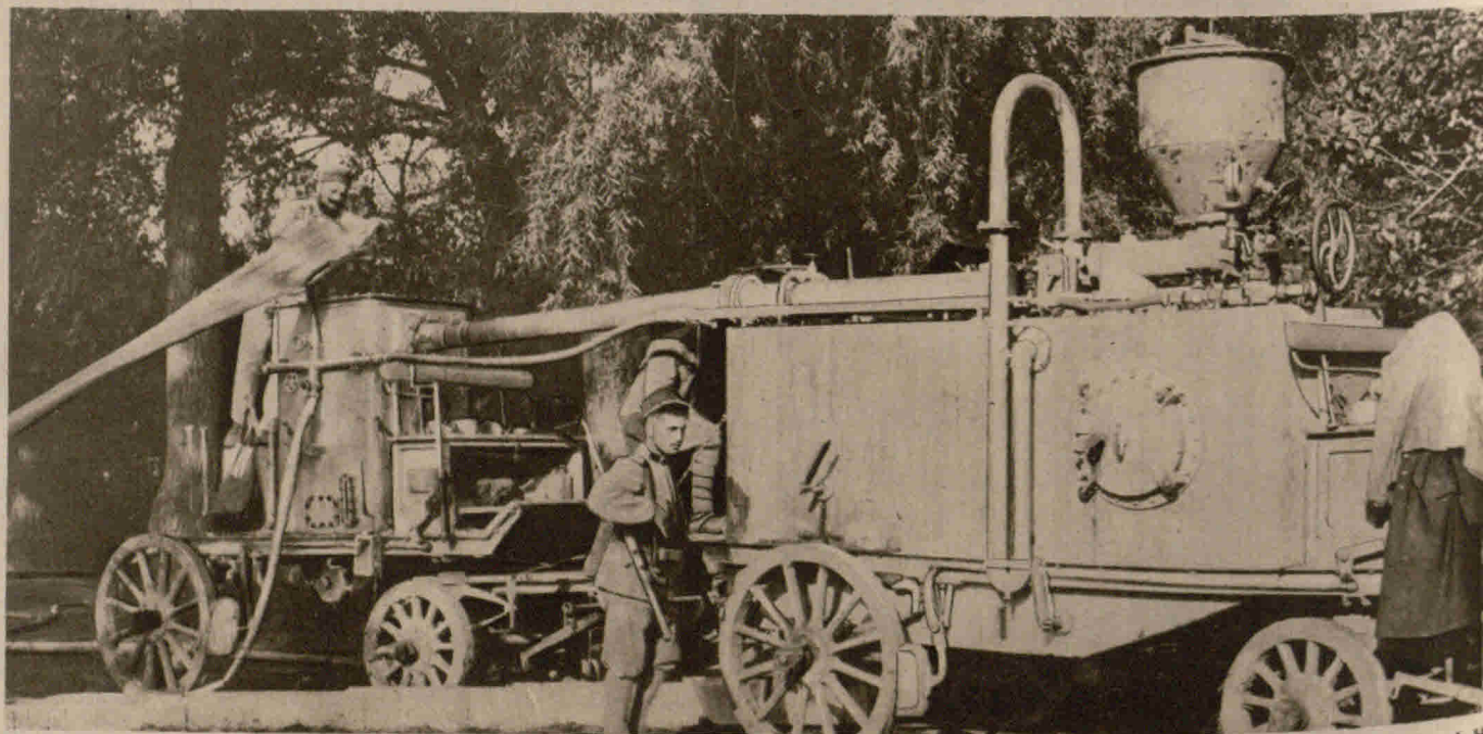
Fahrbarer Apparat zur Erzeugung von Wasserstoffgas für die Füllung von Fesselballons
