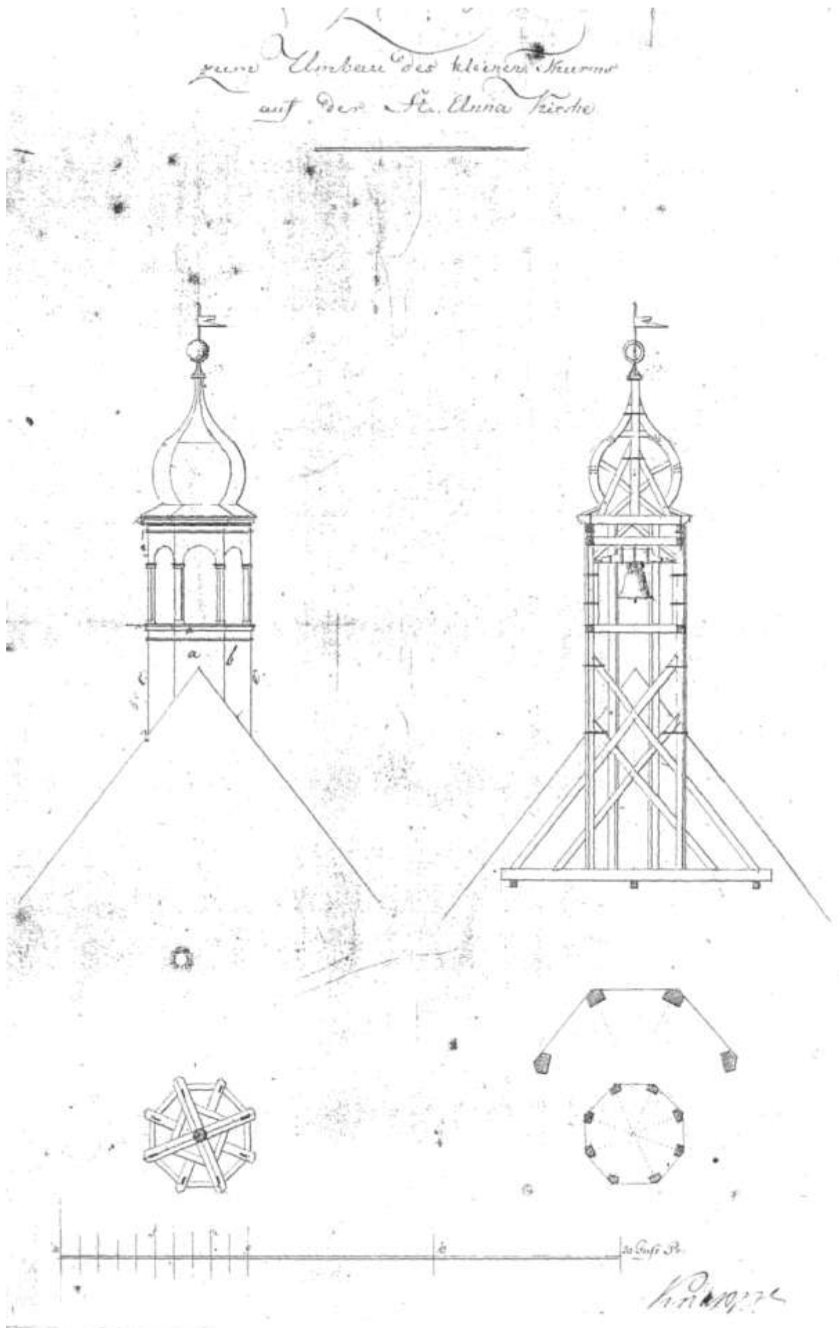
Szkic roboczy wieżyczki kaplicy św. Anny w Jeleniej Górze. Akta miasta Jelenia Góra rys.2874
