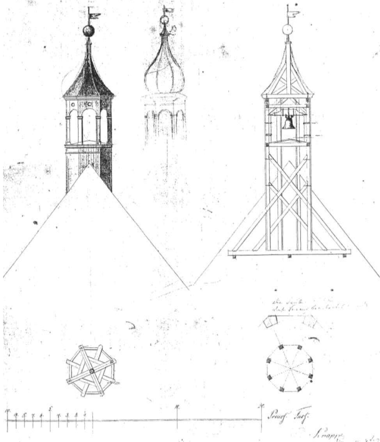
Szkic roboczy wieżyczki kaplicy św. Anny w Jeleniej Górze. Akta miasta Jelenia Góra rys.2874
